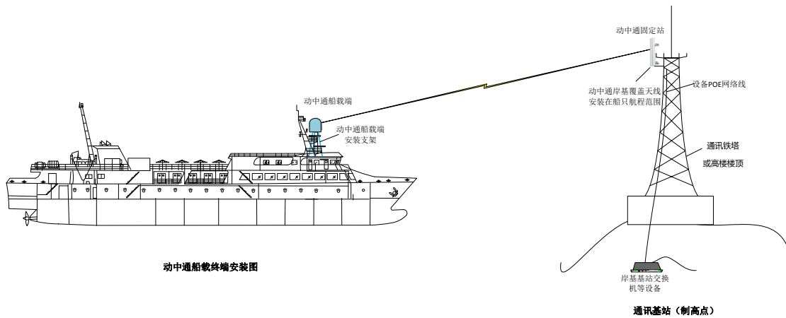
动中通整体系统图
